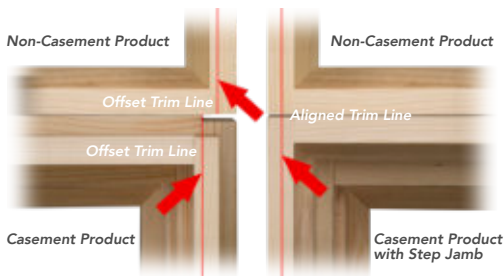
Step Jamb
